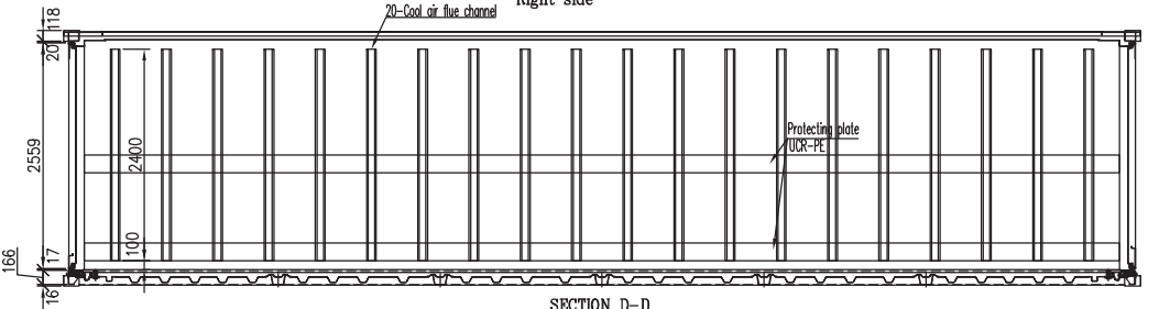
SECTION D-D
